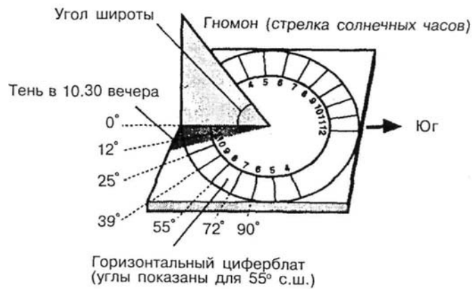
Солнечные часы
