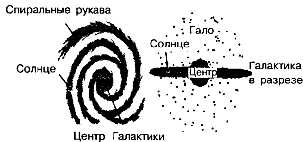
Расположение Солнца
