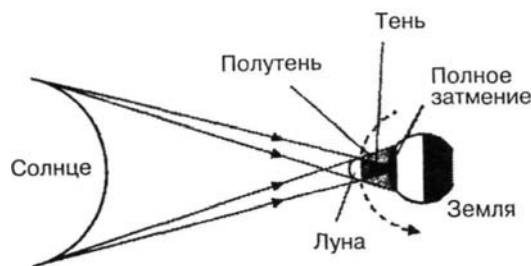
Солнечное затмение
