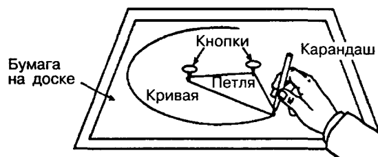
Рисунок эллипса
